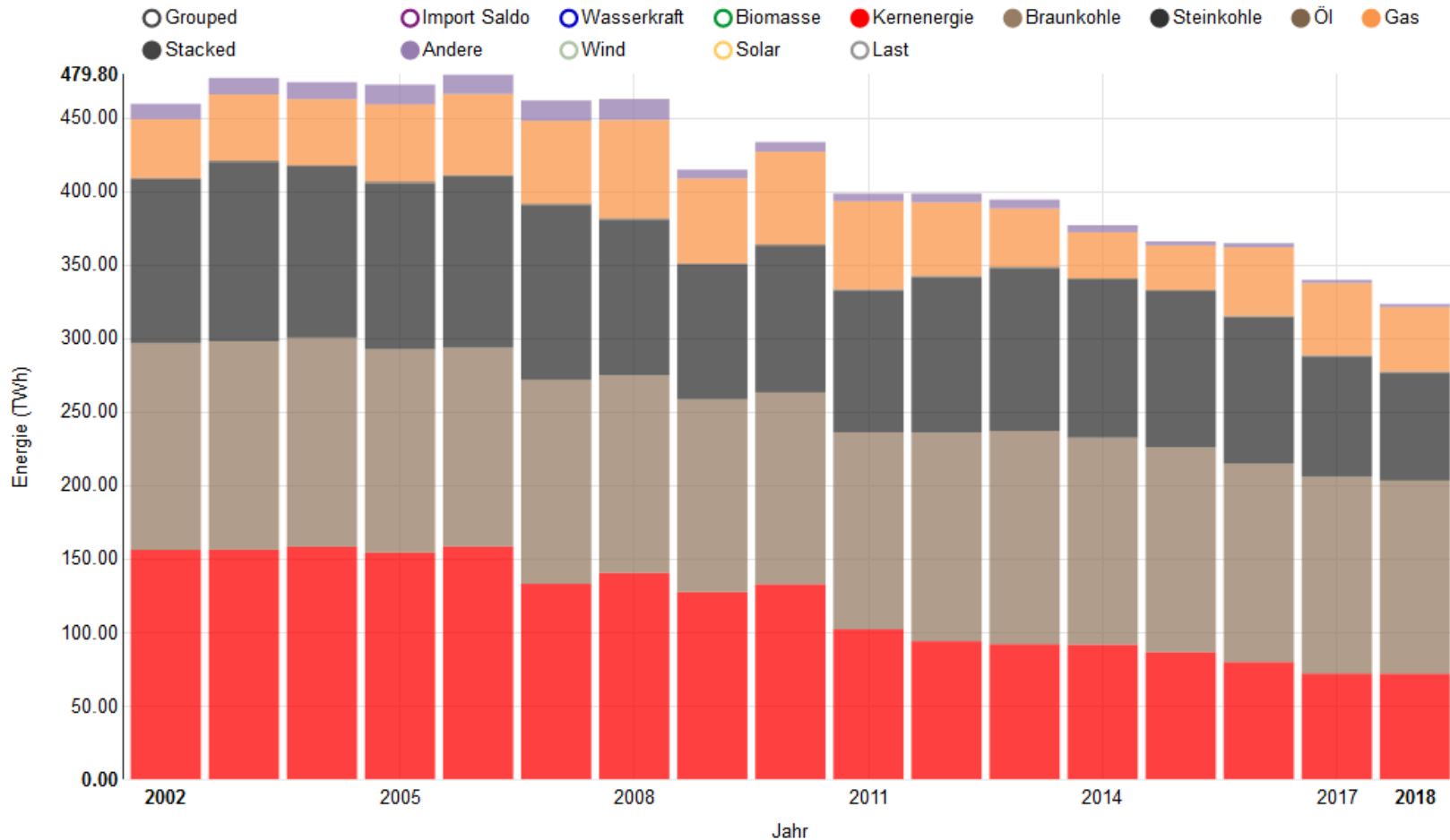
Grafik: B. Burger, Fraunhofer ISE; Quelle: https://www.energy-charts.de/energy_de.htm?source=all-sources
