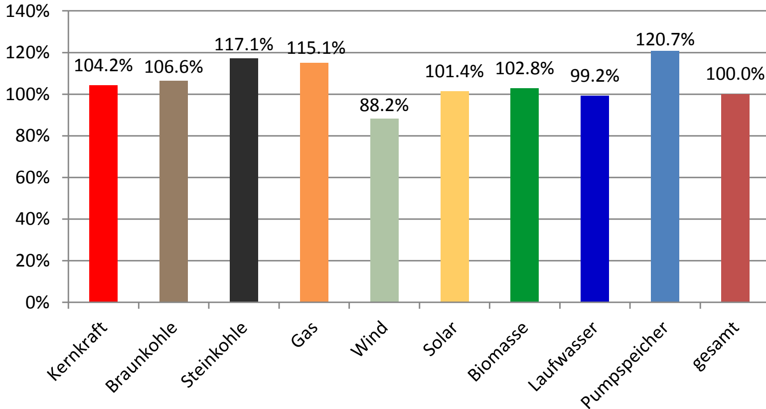
Grafik: B. Burger, Fraunhofer ISE; Daten: EPEX
