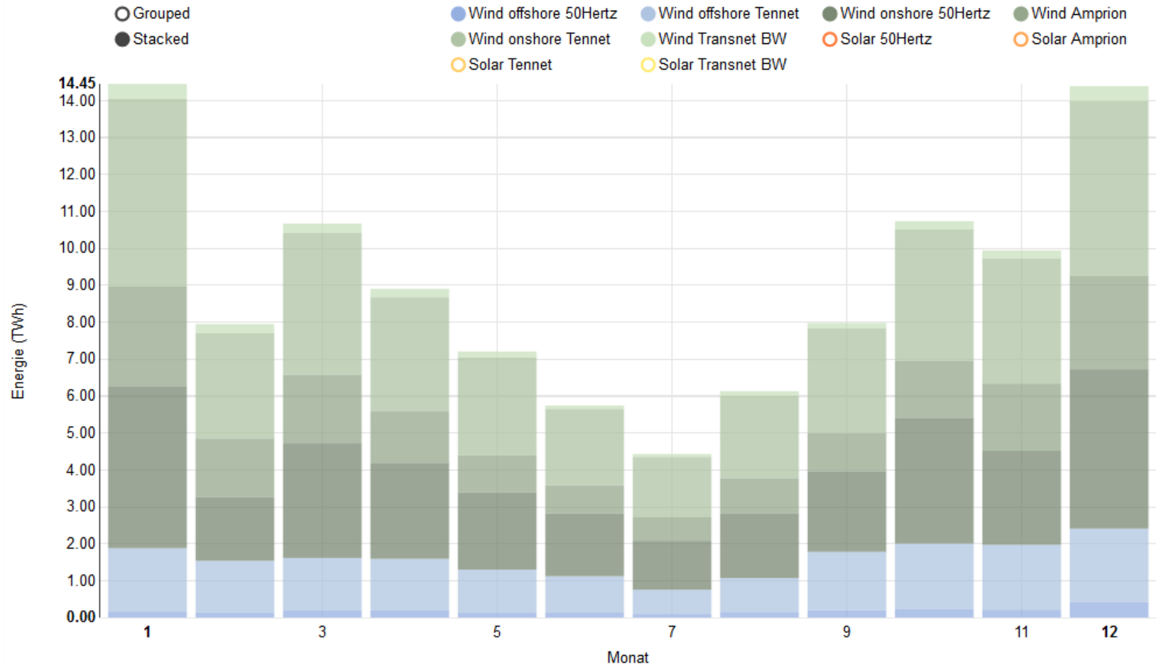
Grafik: B. Burger, Fraunhofer ISE; Quelle: https://www.energy-charts.de/energy_de.htm?source=solar-wind
